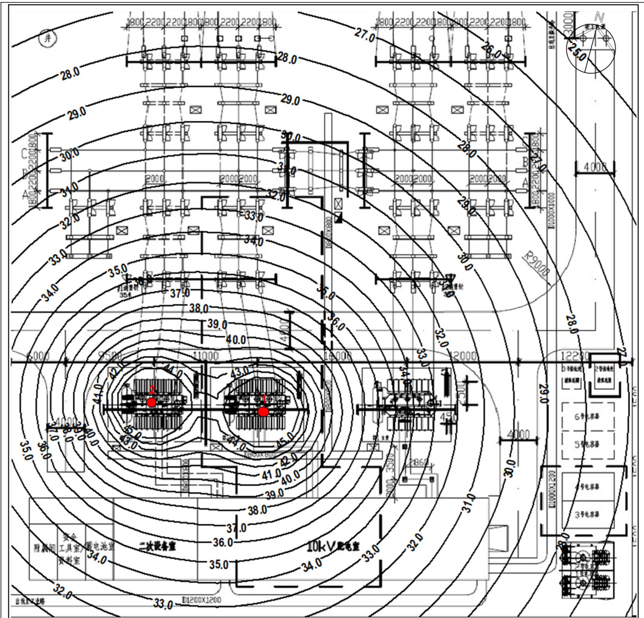
图9 变电站运营期噪声等值线分布图
