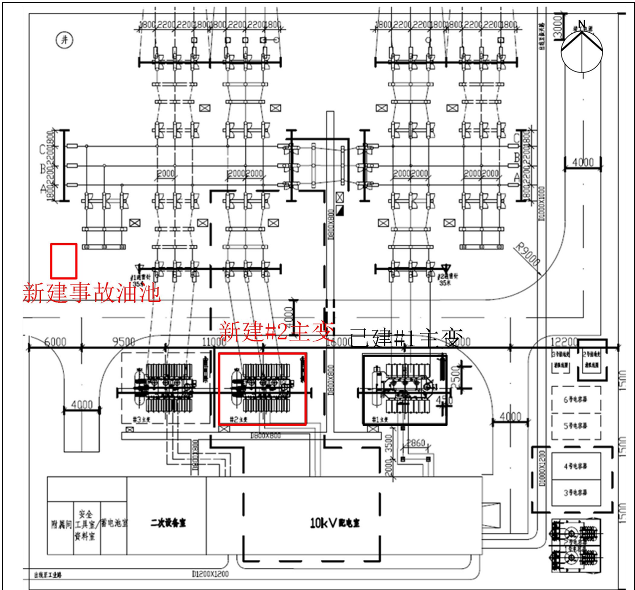
图 2 变电站平面布置图
