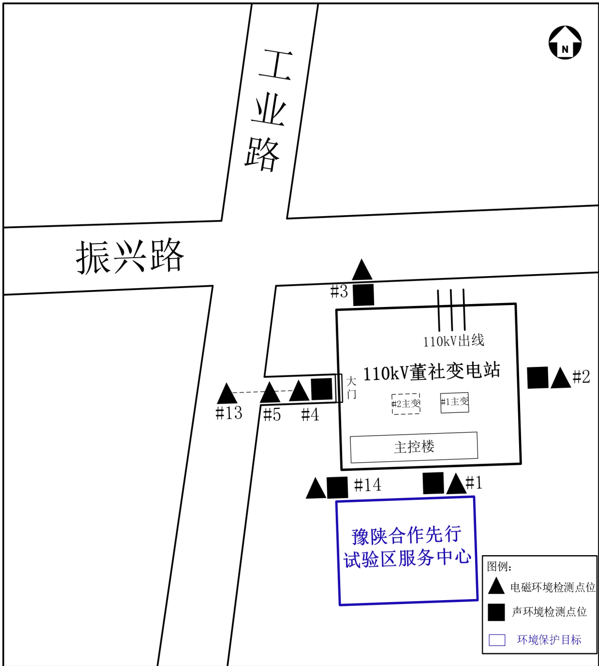
图 5 检测布点示意图
