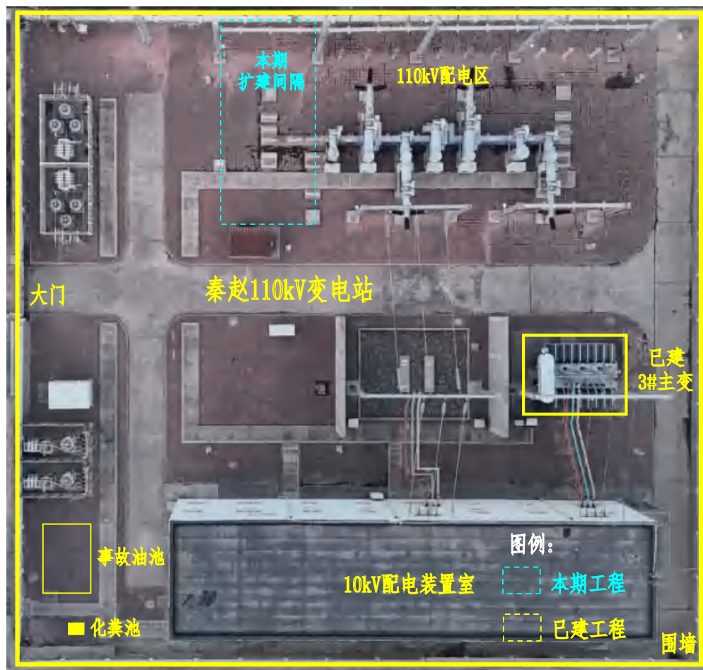
附图09 项目变电站生态环境保护措施总体布局情况示意图
