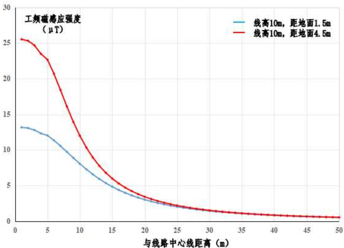
专图 4-3 本项目 110-EC21D-ZM2 典型杆塔单回线路工频电场强度分布曲线
