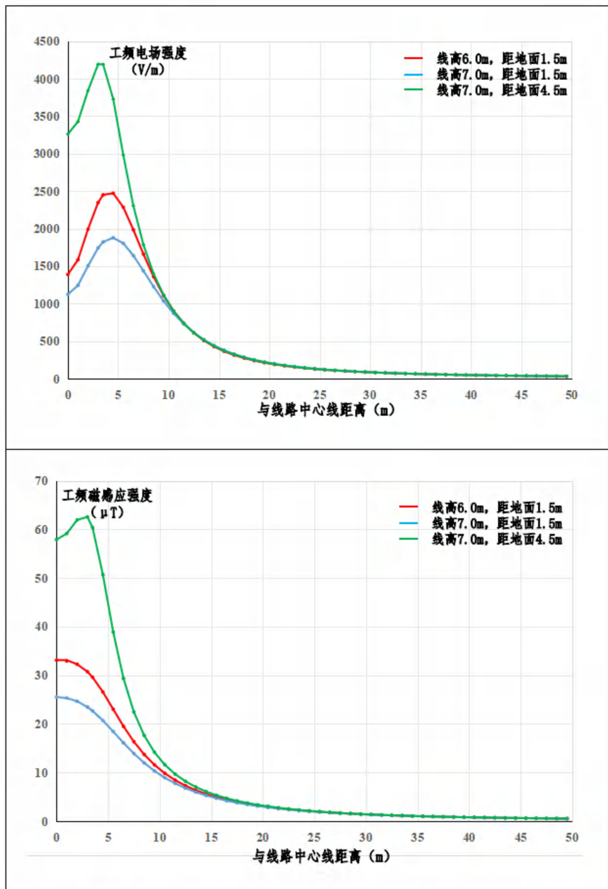
专图 4-1 本项目 110-EC21D-ZM2 典型杆塔单回线路工频电场强度分布曲线
