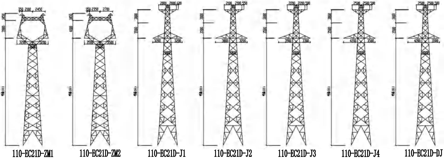
附图01 项目杆塔型式图
