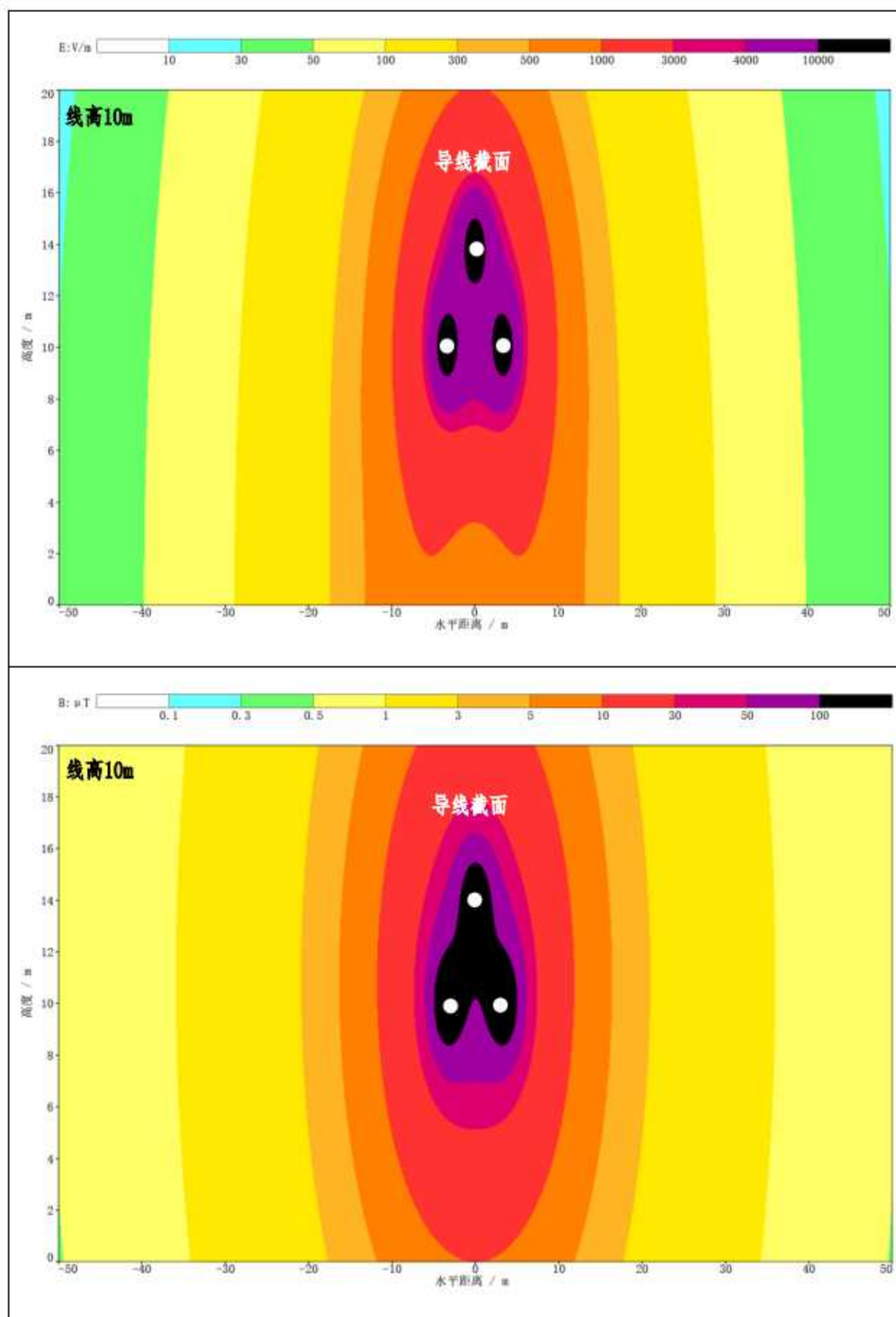
专图 4-4 本项目 110-EG21D-ZM2 典型杆塔单回线路工频电场强度、工频磁感应强度等值线图
