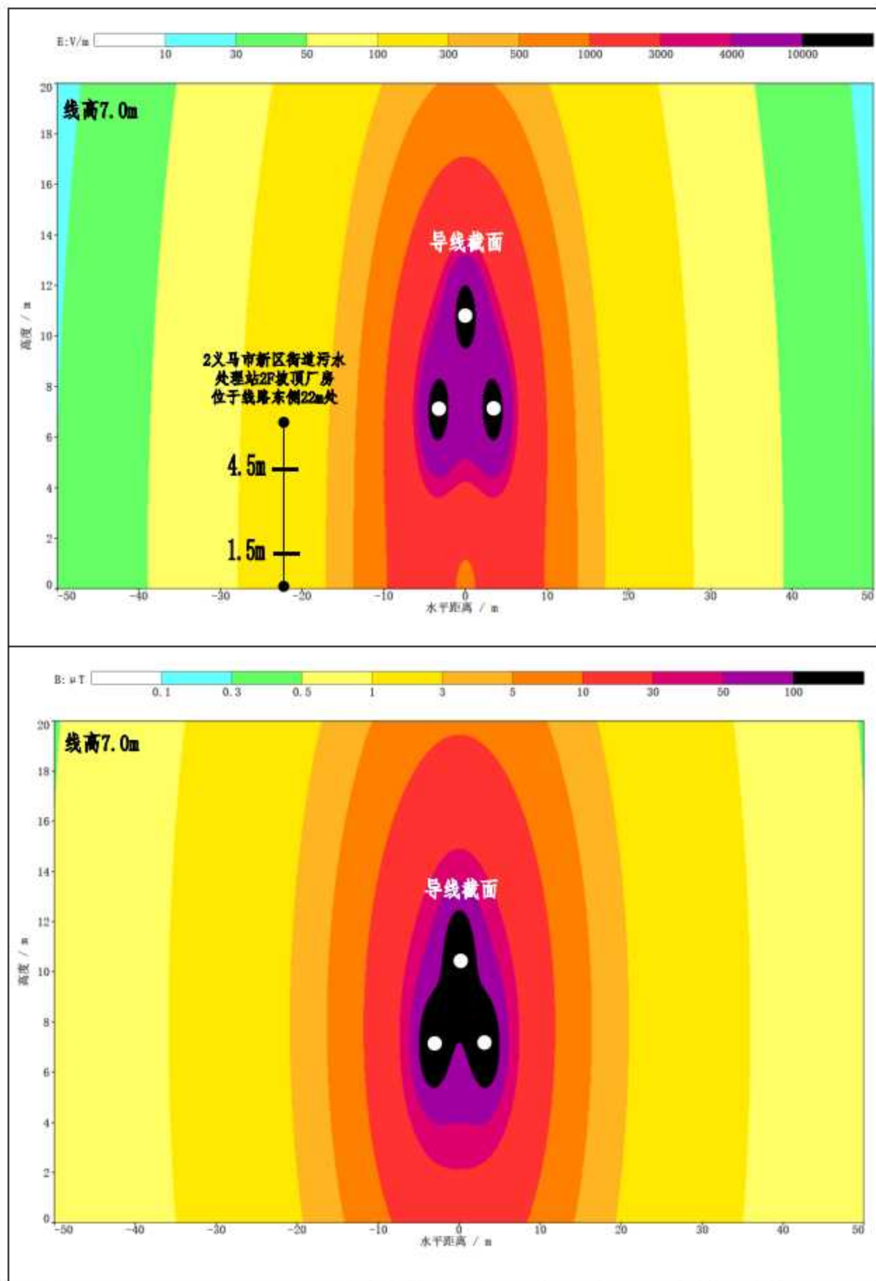
专图 4-2 本项目 110-EG21D-ZM2 典型杆塔单回线路工频电场强度、工频磁感应强度等值线图
