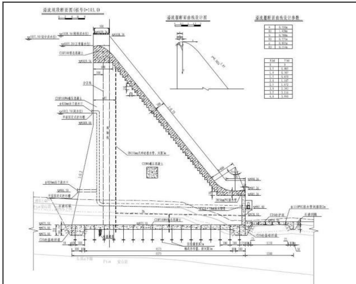
图4.2-7 坝址B剖面图
