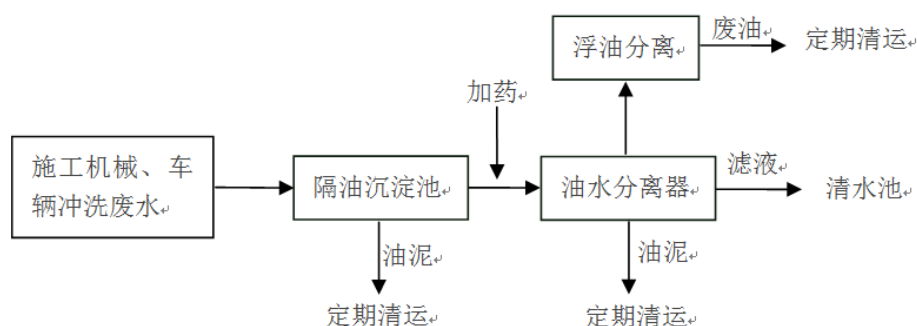
图8.2-3 施工机械、车辆冲洗水处理工艺流程图
