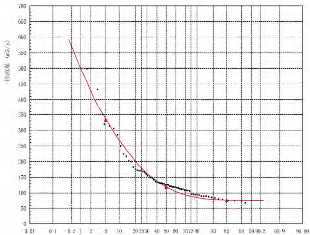
图 5.1-3 竹园沟径流量频率曲线图
