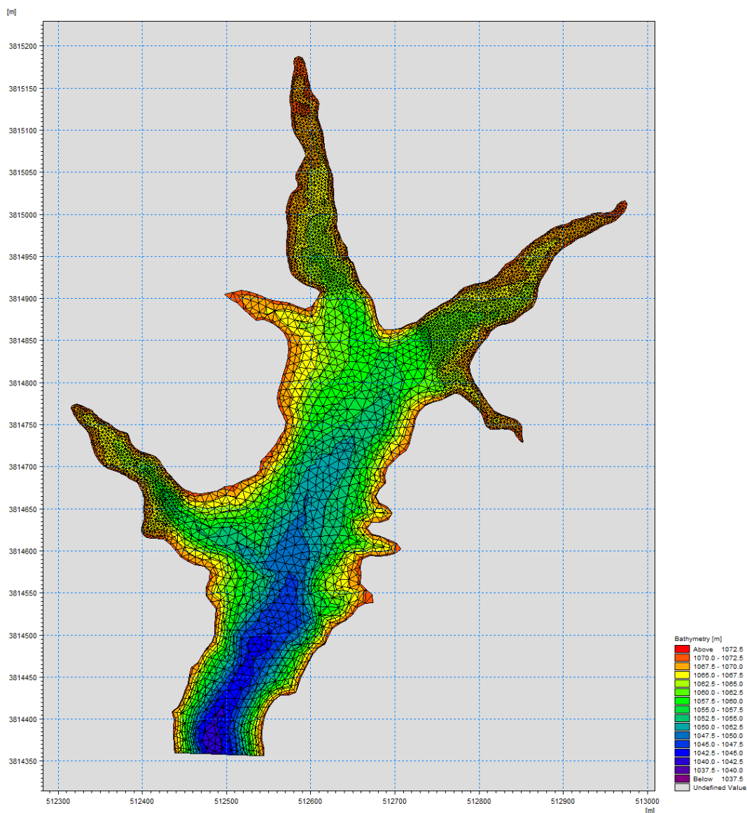
图7.1-14 本次评价区库区整体地形高程图
