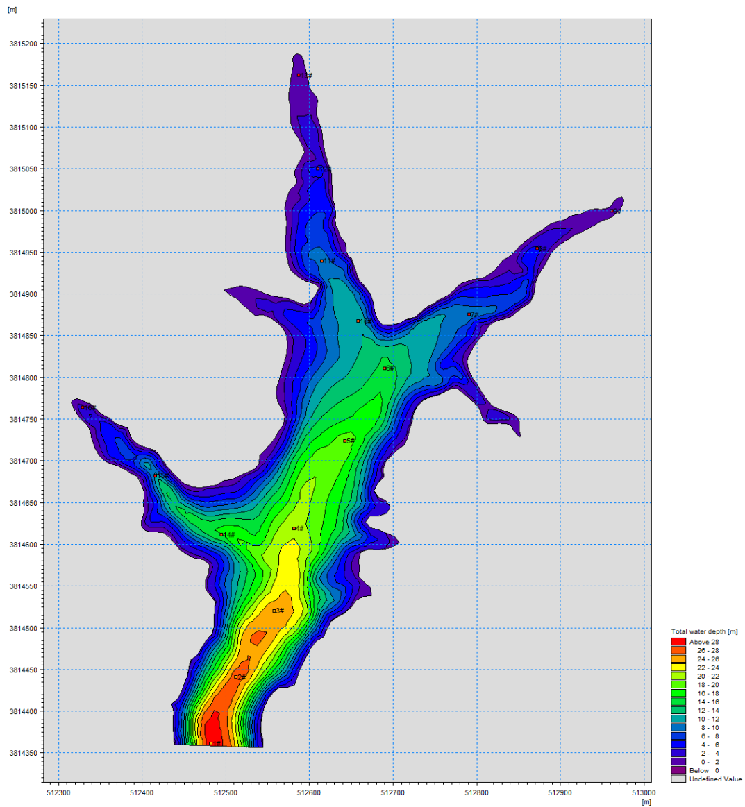
图7.1-20 丰水期10%保证率下流量对应的库区水深 表7.1-13 工程后库区枯、丰水期观测点处水深对比表
