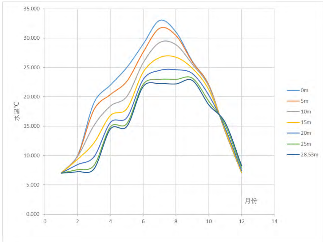
图7.1-25 水库水温~月份关系曲线图
