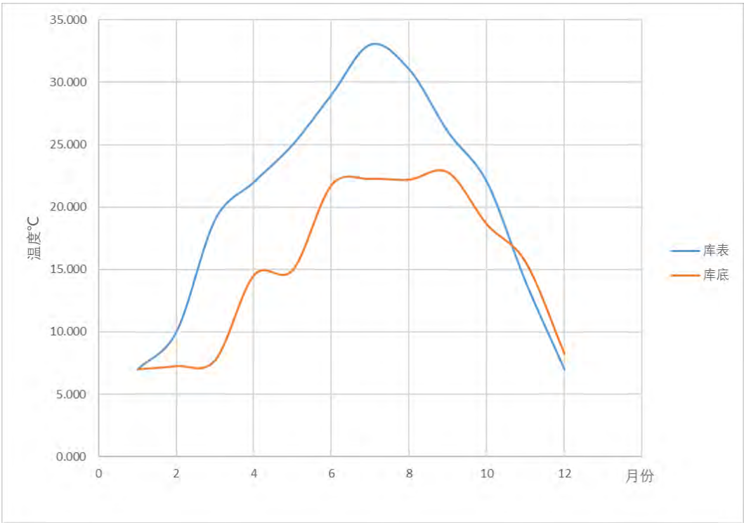
图7.1-27 水库库表及库底水温关系曲线图
