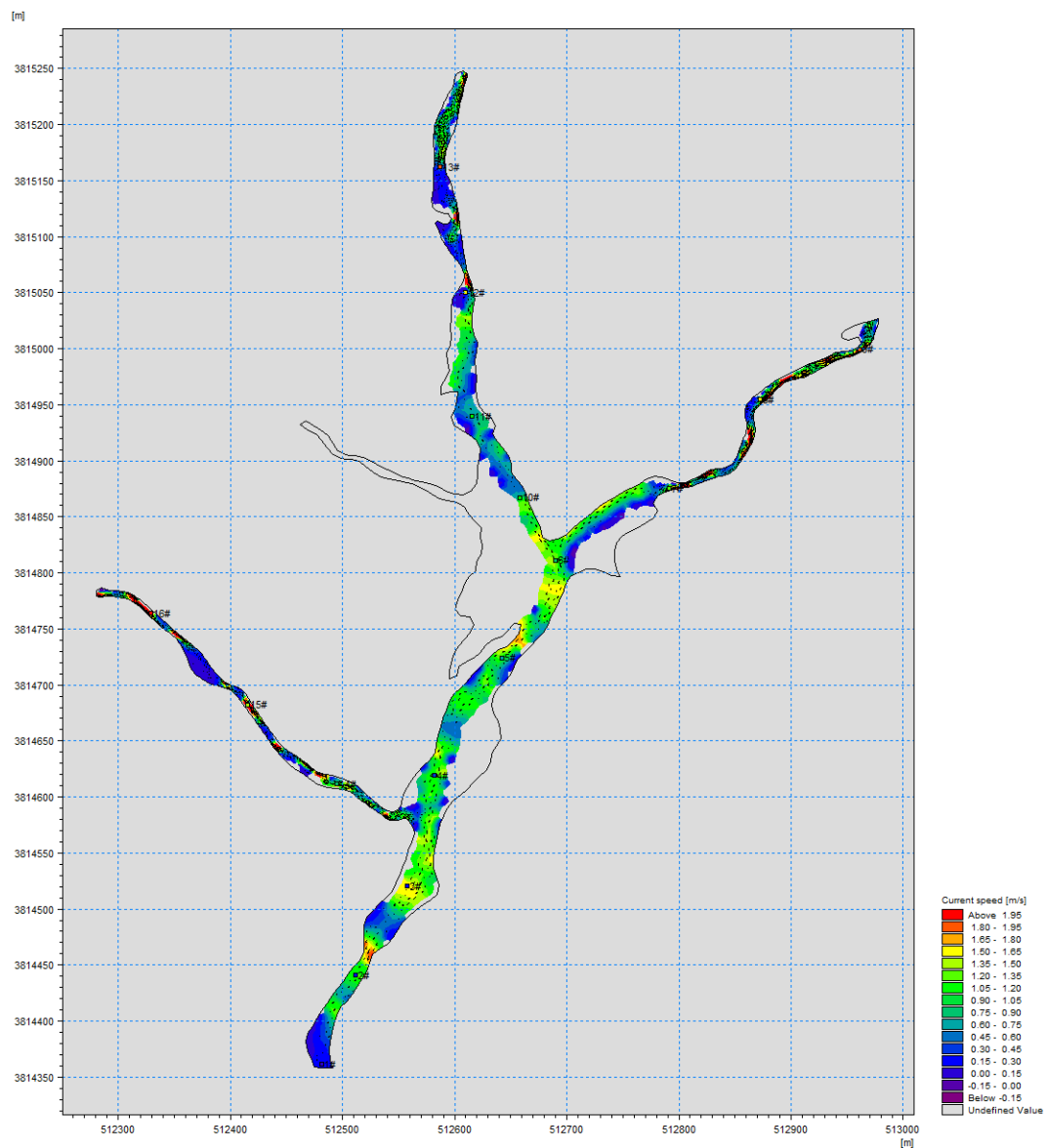
图7.1-10 丰水期10%保证率下流量对应的河流流速 表7.1-9 现状河流枯、丰水期观测点处流速对比表
