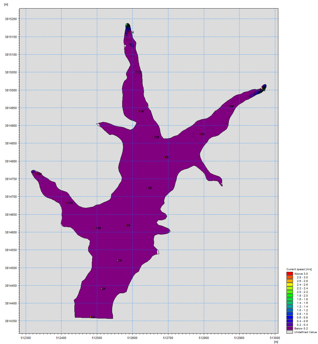
图7.1-22 丰水期10%保证率下流量对应的库区流速 表7.1-14 工程后库区枯、丰水期观测点处流速对比表
