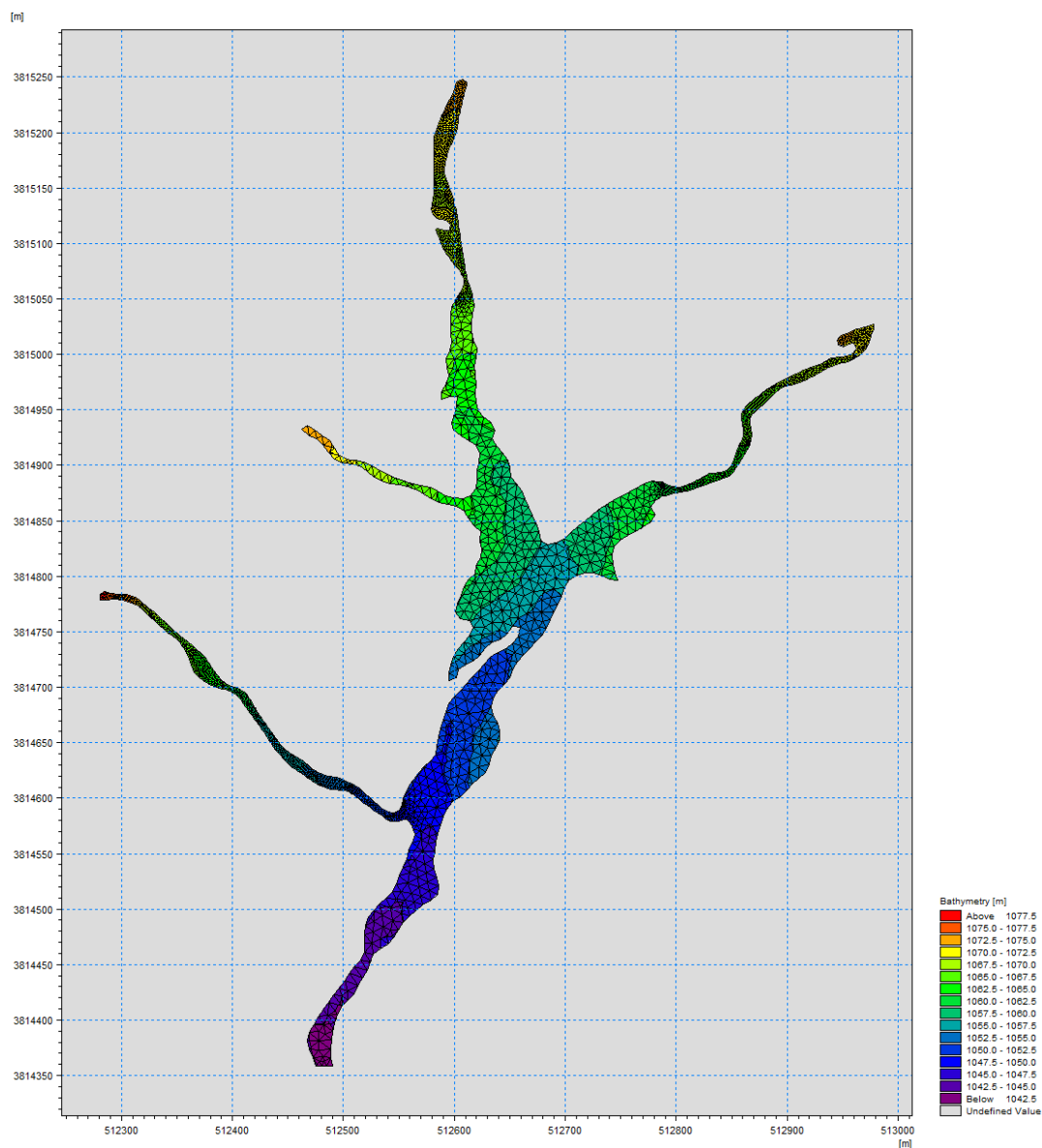
图7.1-2 本次评价区现状河流地形高程图
