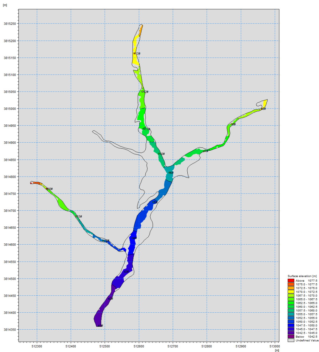
图7.1-5 枯水期90%保证率下流量对应的河流水位
