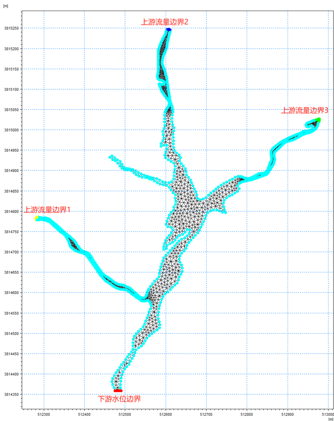
图7.1-3 评价区现状河流边界设置图
