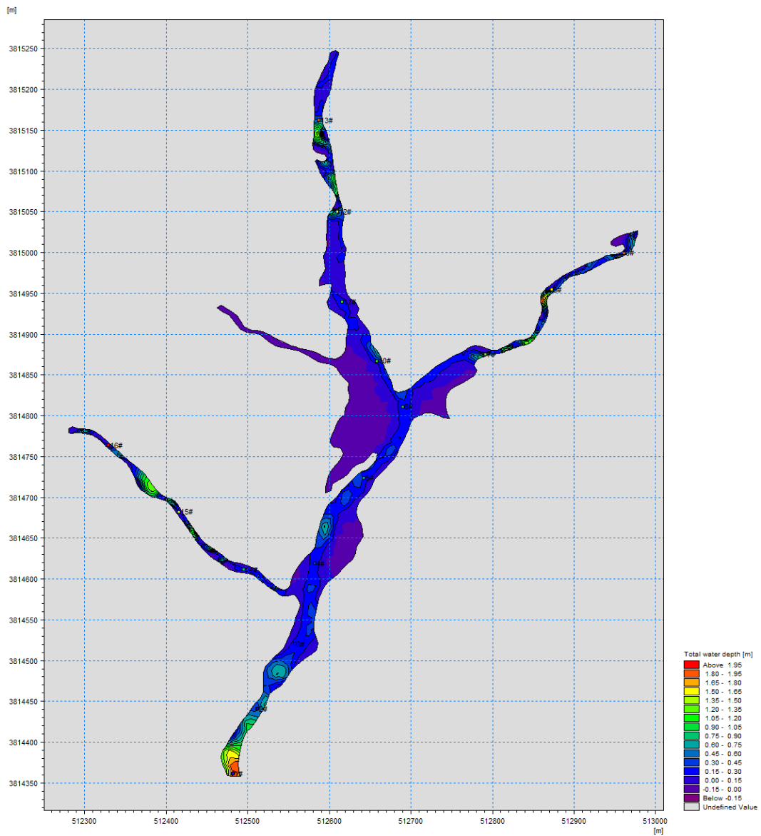
图7.1-8 丰水期10%保证率下流量对应的河流水深 表7.1-8 现状河流枯、丰水期观测点处水深对比表
