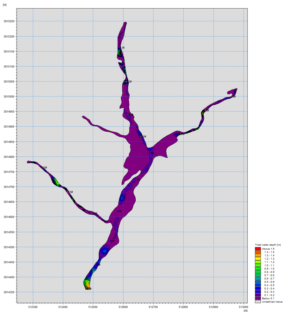
图7.1-7 枯水期90%保证率下流量对应的河流水深
