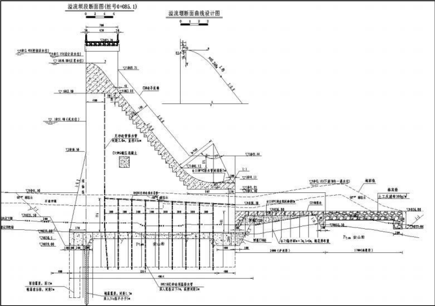
图4.2-10 坝线B剖面图
