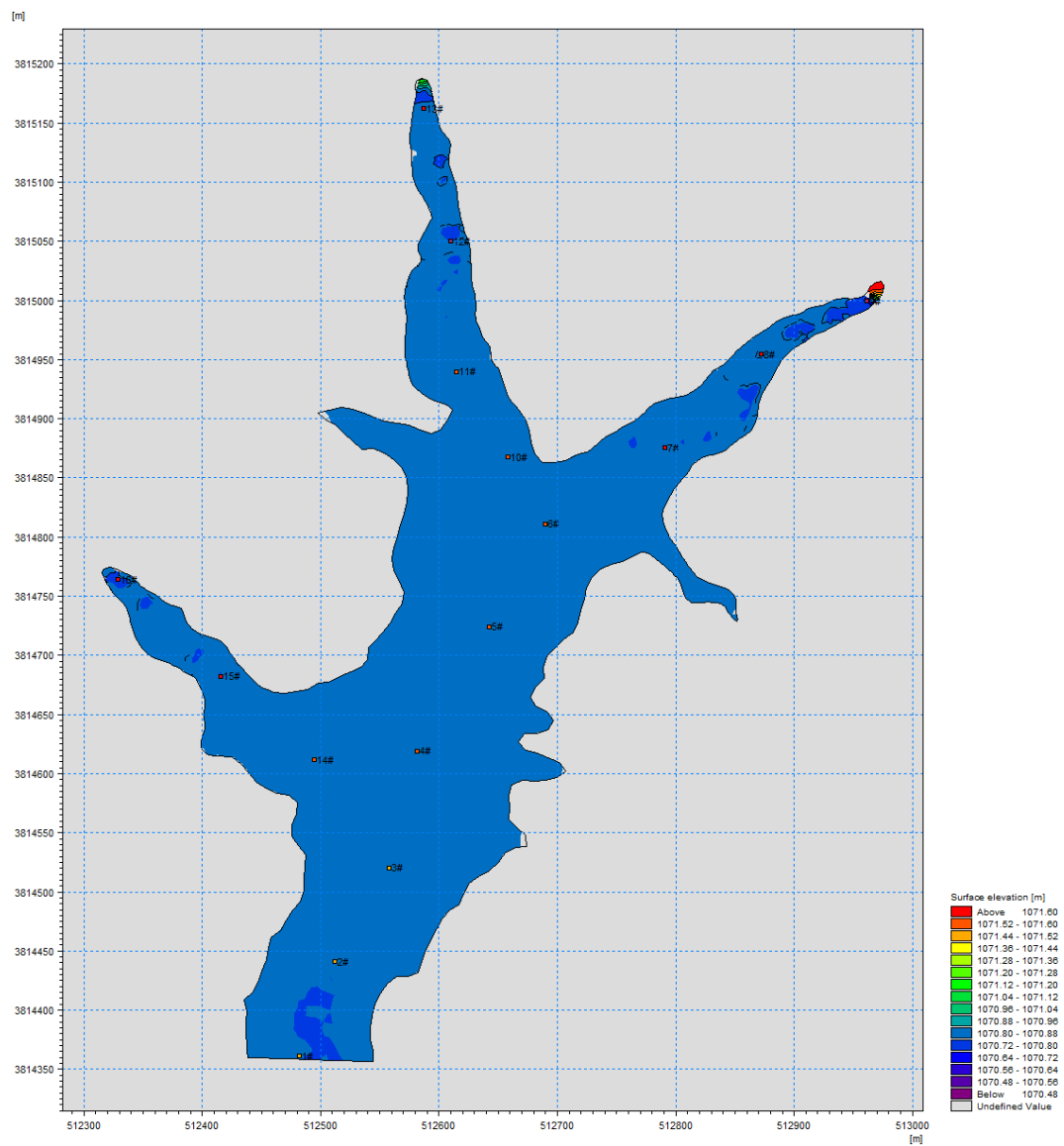
图7.1-18 丰水期10%保证率下流量对应的库区水位 表7.1-12 工程后库区枯、丰水期观测点处水位对比表
