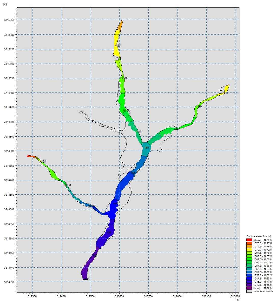
图7.1-6 丰水期10%保证率下流量对应的河流水位 表7.1-7 现状河流枯、丰水期观测点处水位对比表
