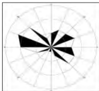
图5.1-1 近20年全年风向玫瑰图
