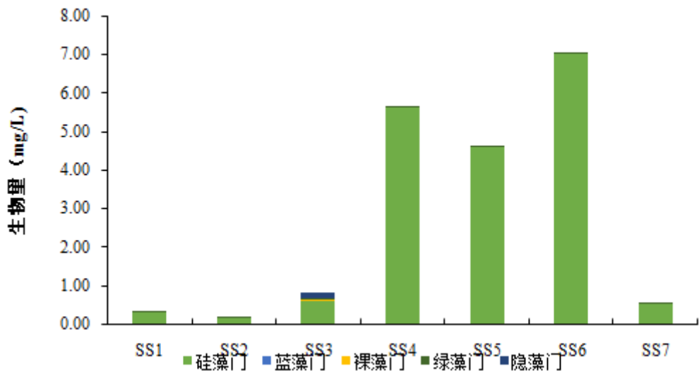
图5.6-6 各样点浮游植物生物量分布图
