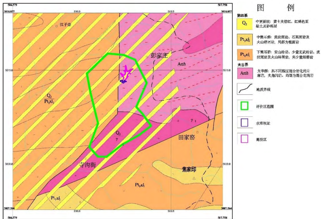
图7.2-2 评价区地质图
