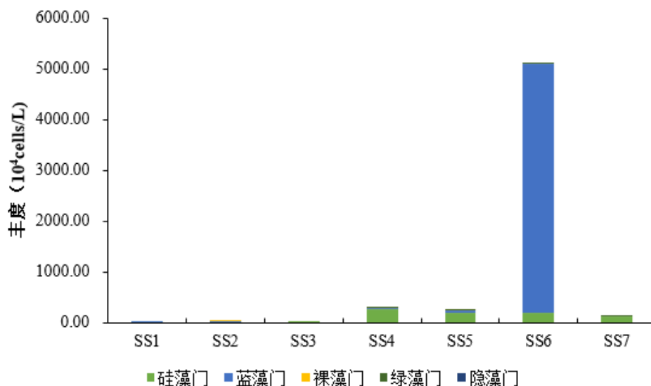
图5.6-7 各样点浮游植物丰度分布图
