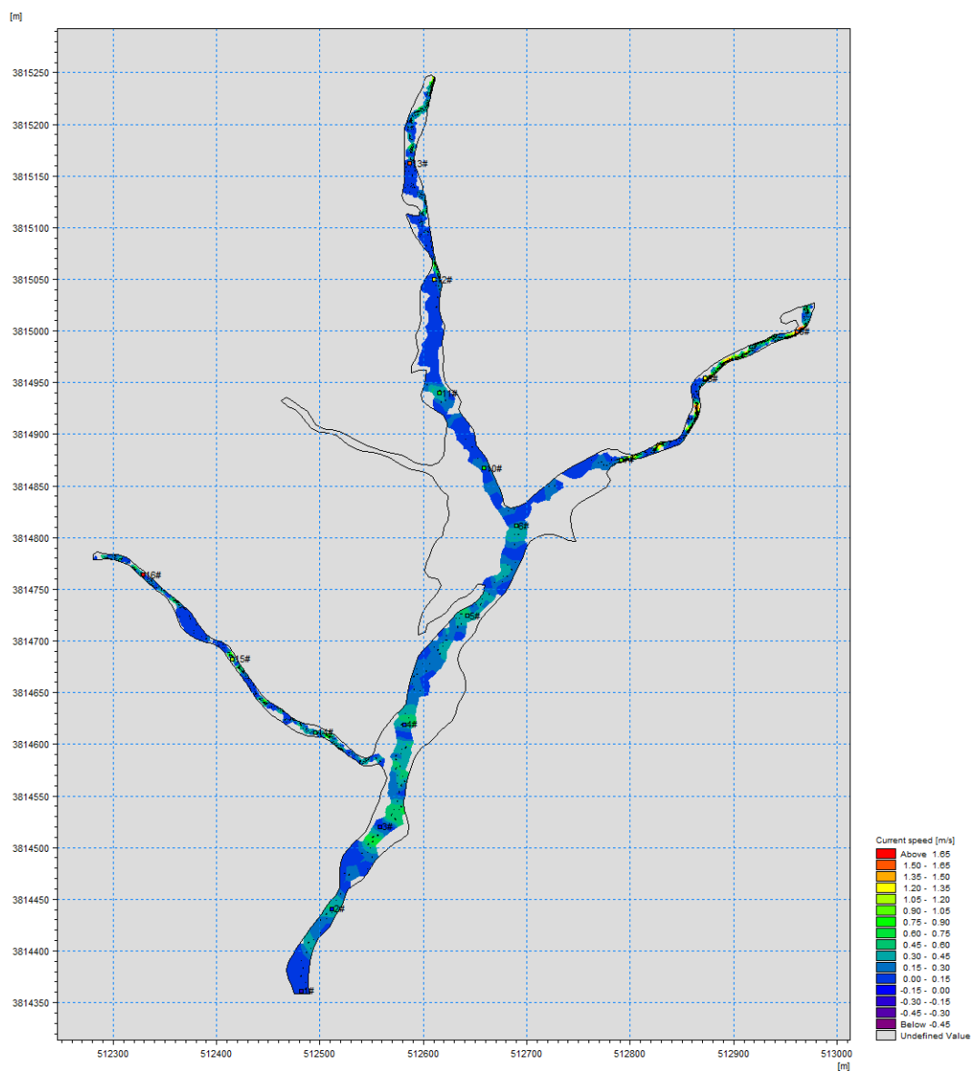
图7.1-9 枯水期90%保证率下流量对应的河流流速
