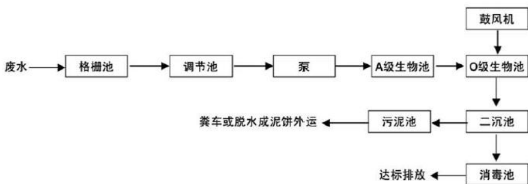
图8.2-1 一体化生活污水处理工艺流程图
