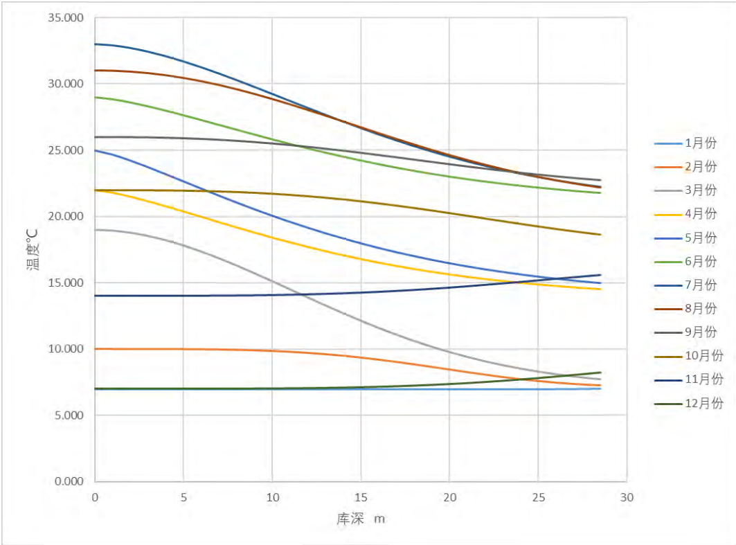
图7.1-26 水库水温~水深关系曲线图
