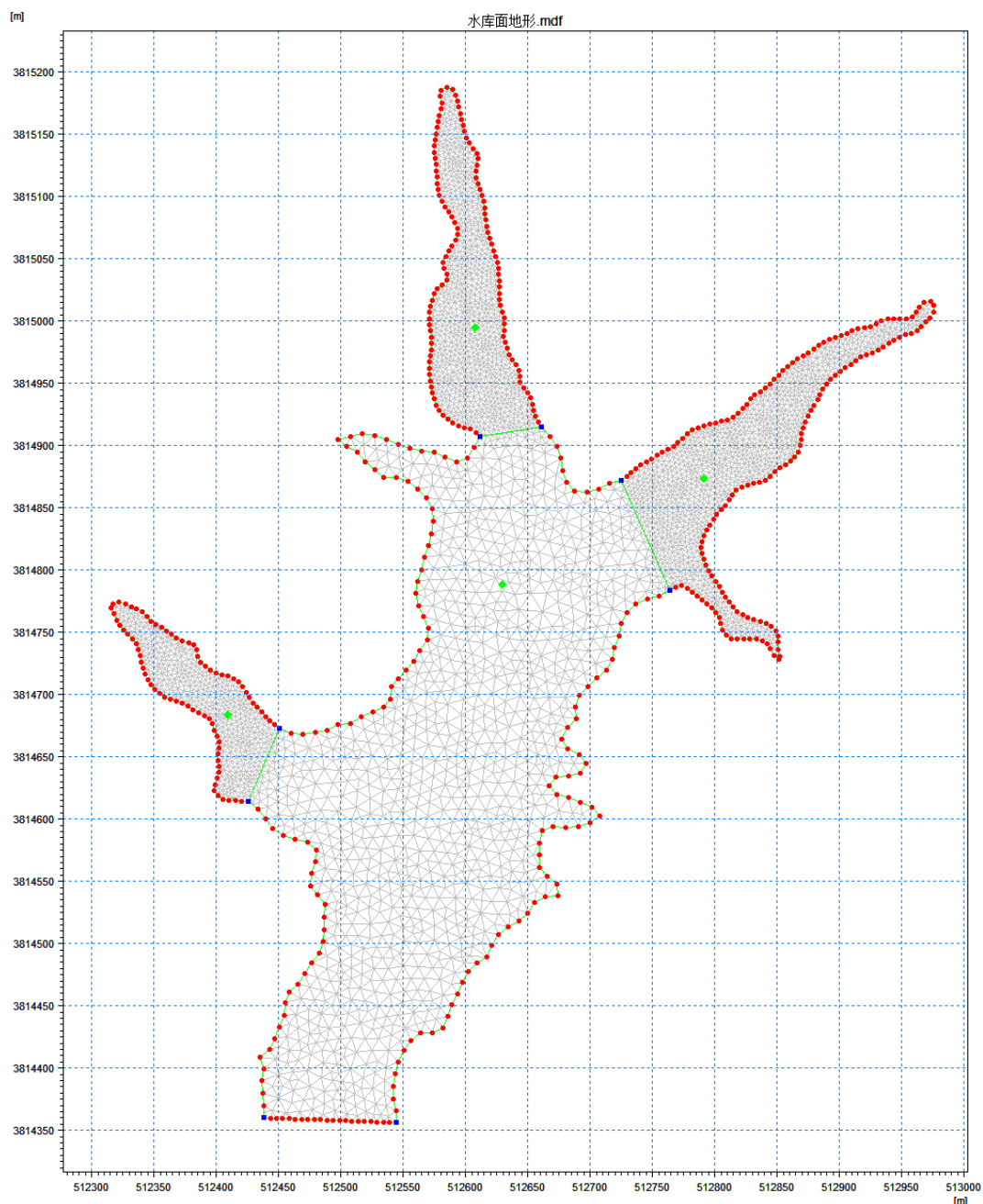
图7.1-13 本次评价区库区网格剖分图
