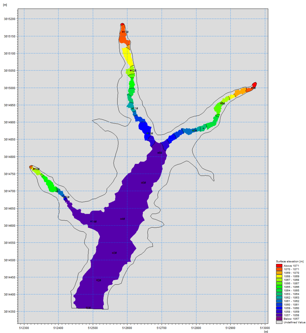
图7.1-17 枯水期90%保证率下流量对应的库区水位
