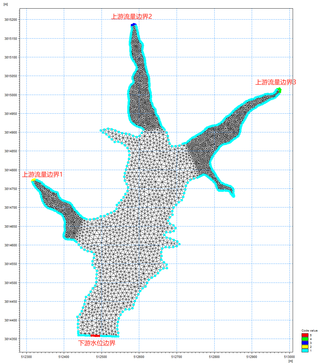
图7.1-15 评价区边界设置位置图
