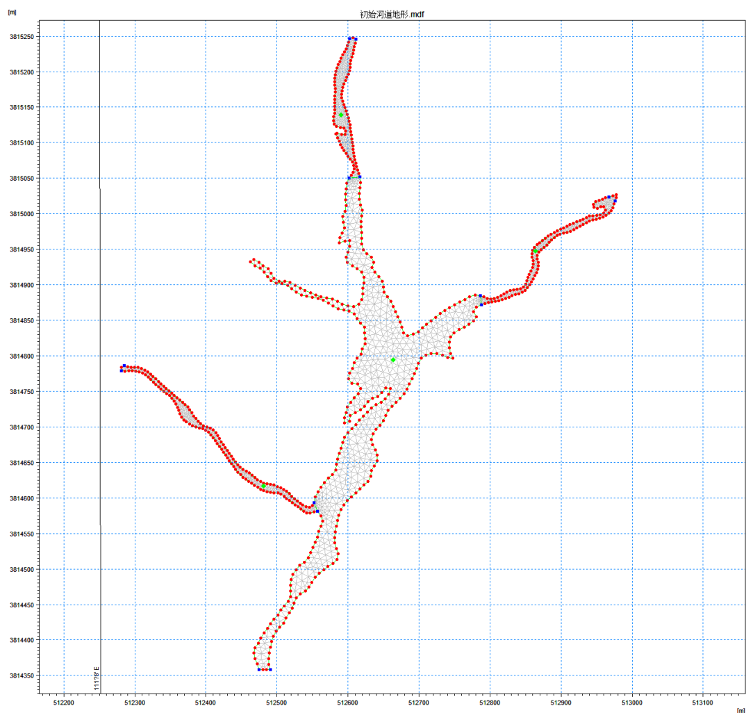
图7.1-1 现状评价区河段网格剖分图
