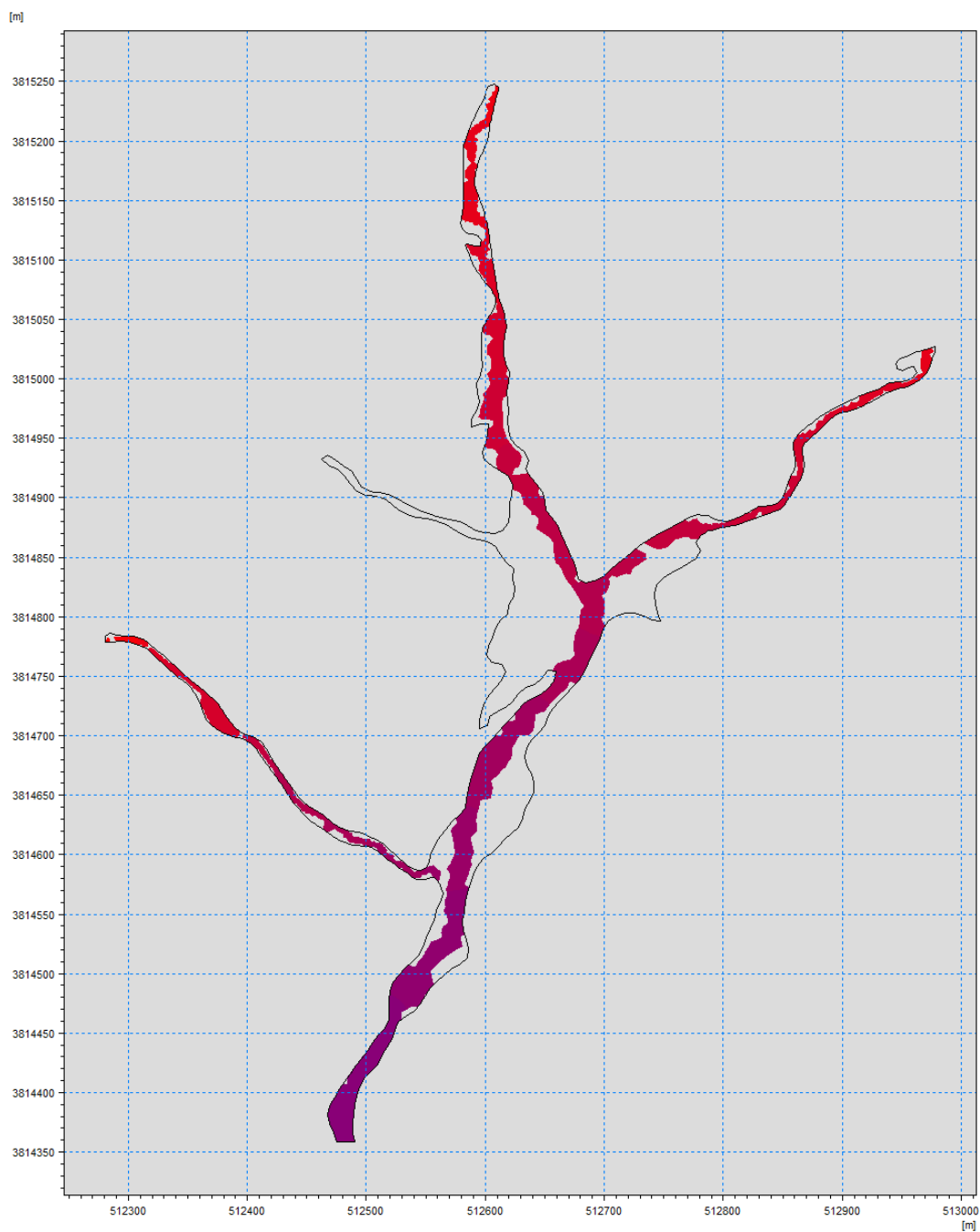
图7.1-11 枯水期90%保证率下流量对应的河流水域面
