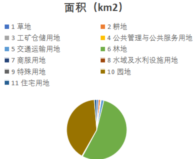
图5.5-1 土地利用类型图
