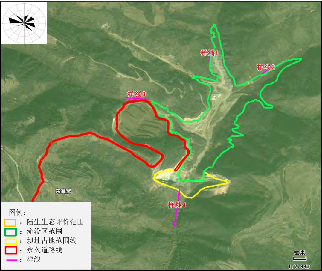
图5.5-6 生态评价范围调查样线图
