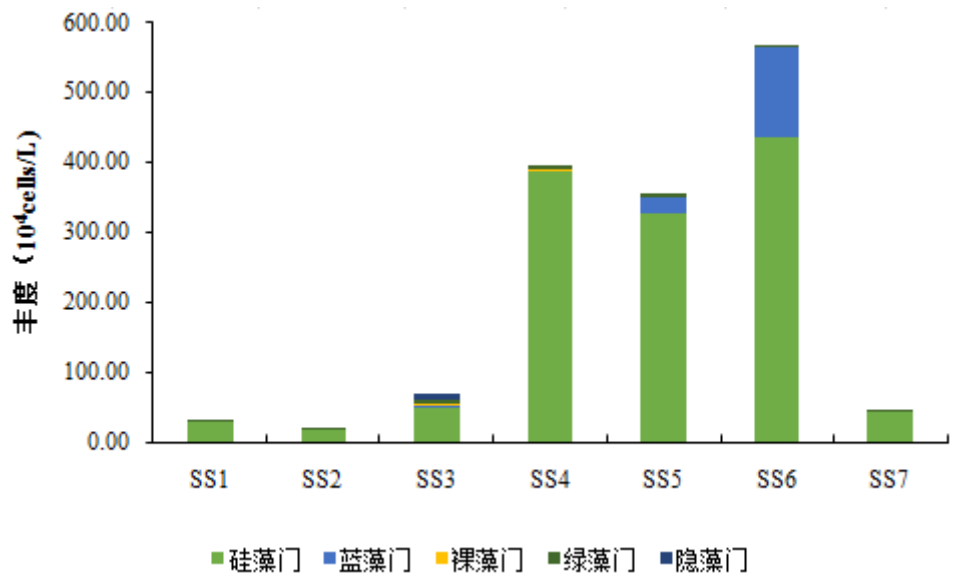
图5.6-5 各样点浮游植物丰度分布图
