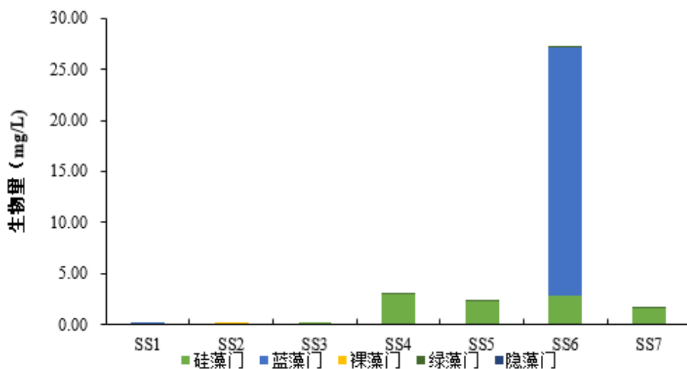
图5.6-8 各样点浮游植物生物量分布图
