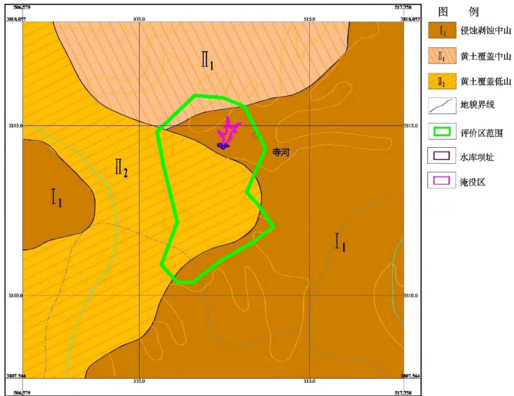
图7.2-1 评价区地貌图
