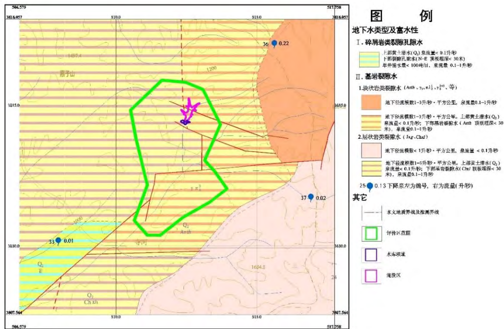
图7.2-3 评价区水文地质图
