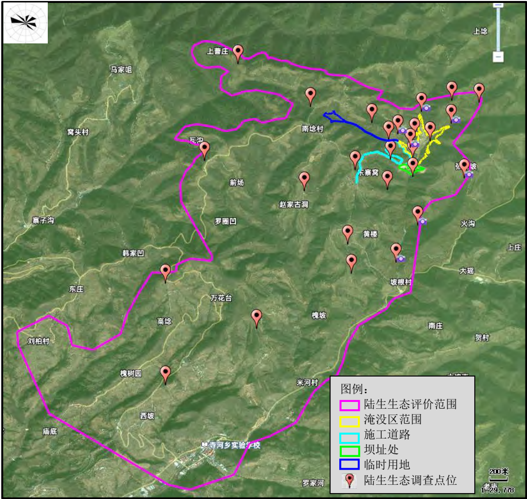
图5.5-2 生态调查样方位置图 样方调查照片见下图。
