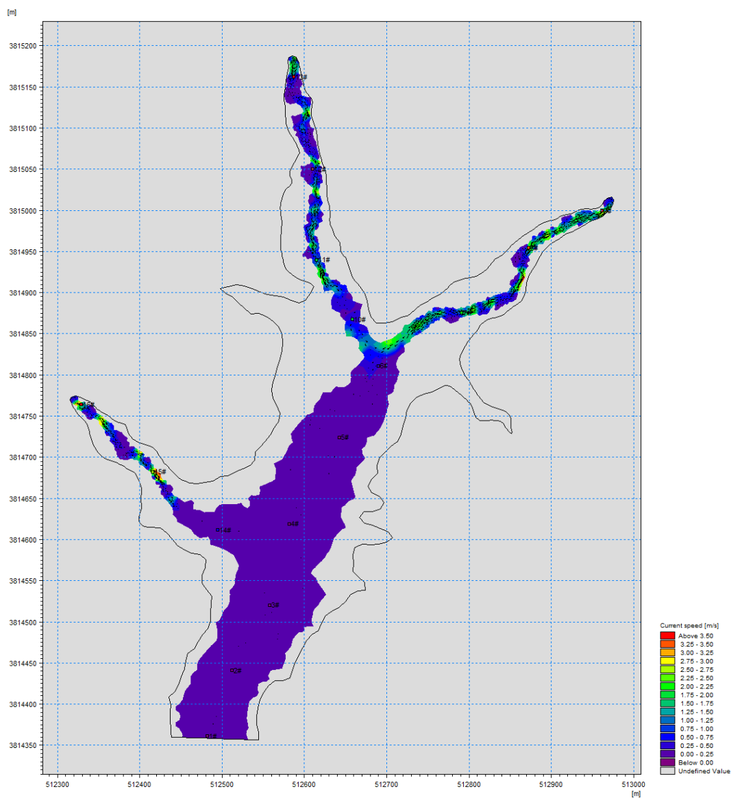
图7.1-21 枯水期90%保证率下流量对应的库区流速
