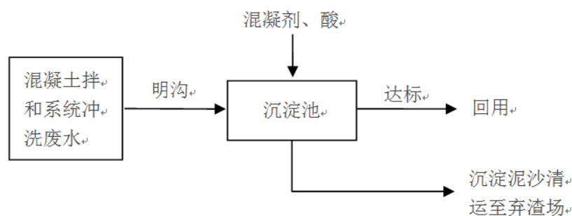
图8.2-2 混凝拌和系统冲洗废水处理工艺流程图
